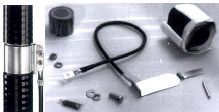
Kit Standard: Cabo de aterramento 610mm
