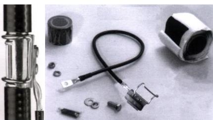
Kit SureGround Instalação mais rápida e prática. Cabo de aterramento 600 e 1200 mm
